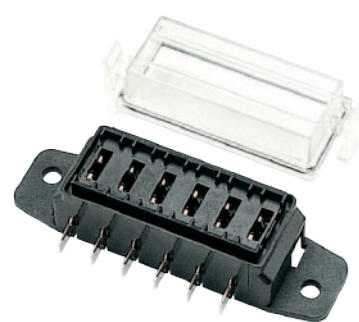
201-06MT 6 Way Mini Fuse Block
