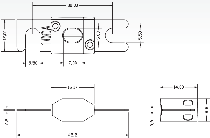
Scale : mm
