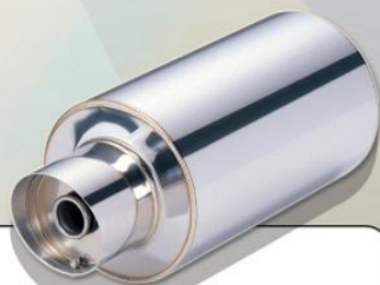
CR-7531T Ø63.5m/m(Ø2-1/2") Tip:SO-115RS Slant
