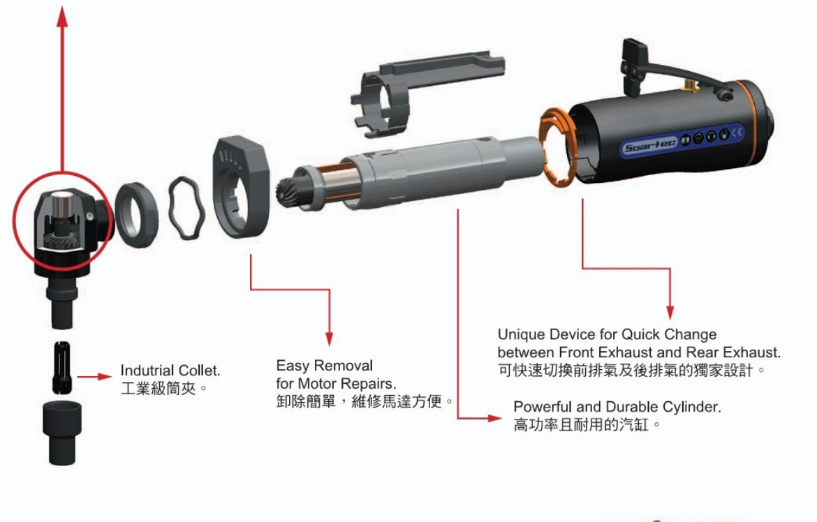
Our Particular Gear Set 曙翔特殊齒輪組
