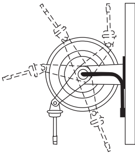
可換向 Switching
