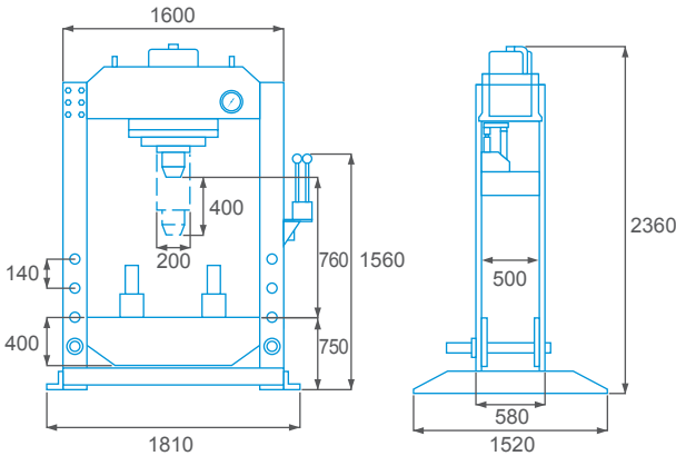
尺寸圖 Dimension
