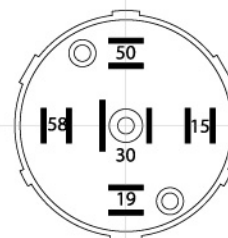
Lid - Terminals
